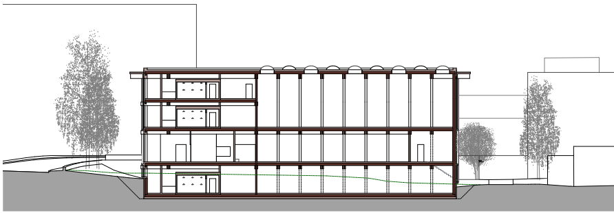
Längsschnitt
