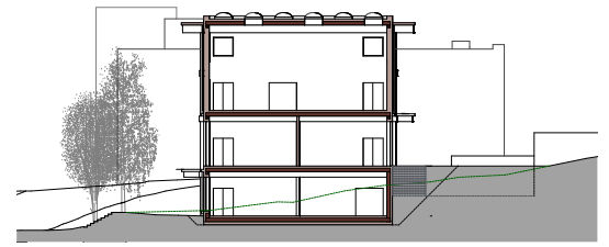
Querschnitt
