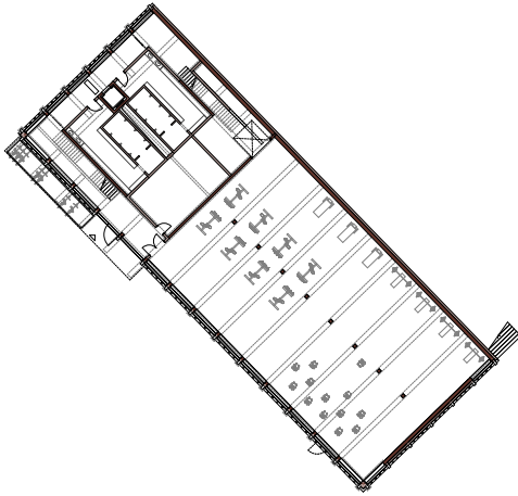
Grundriss Sockelgeschoss
