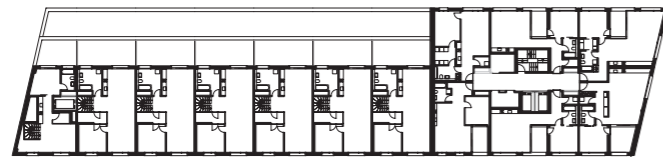
NIVEAU +8 | 8. OBERGESCHOSS
