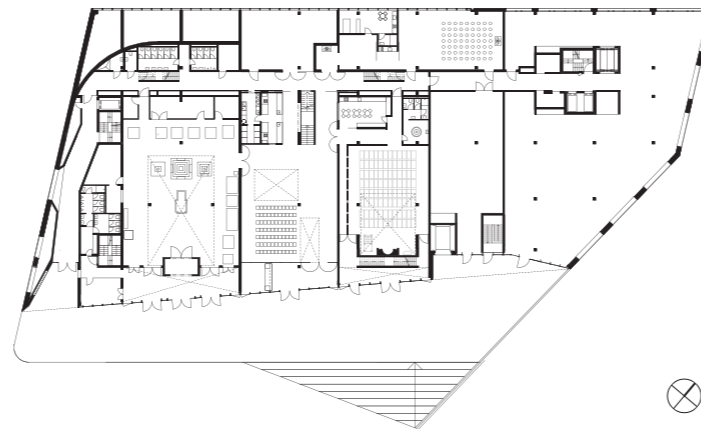
NIVEAU +1 MAISON DES RELIGIONS | 1. OBERGESCHOSS HAUS DER RELIGIONEN
