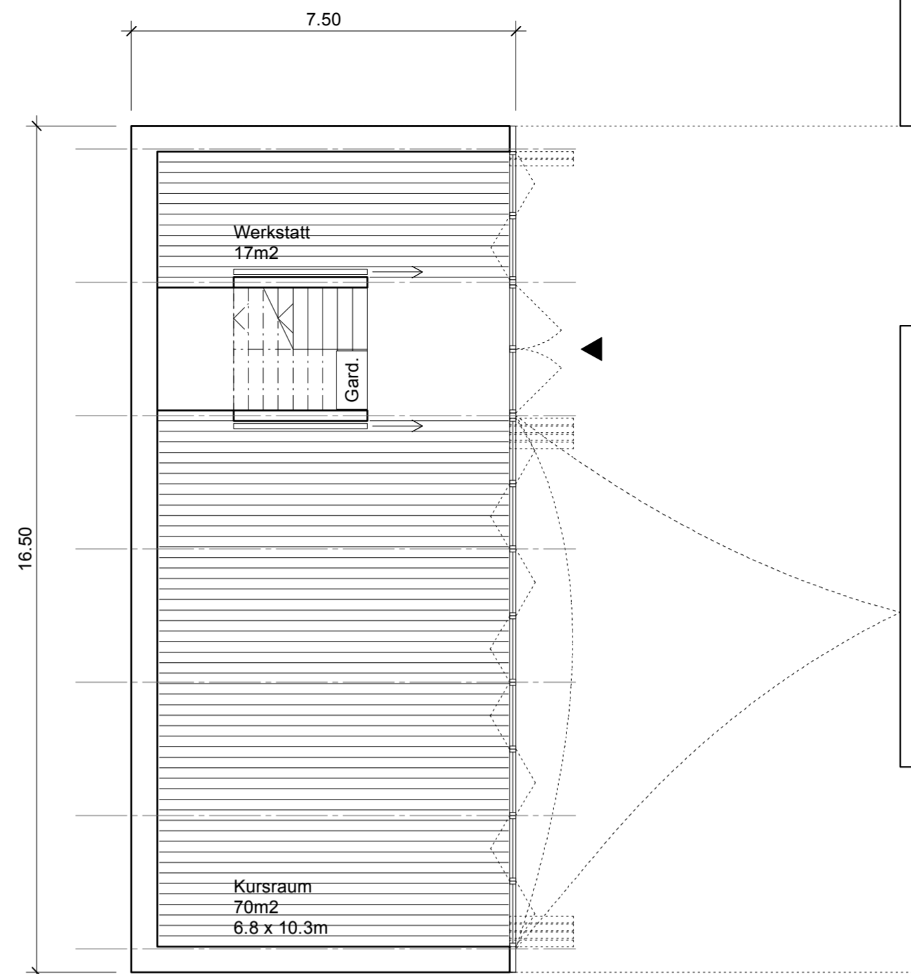
Grundriss Erdgeschoss
