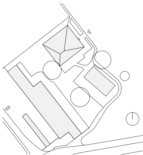
Lageplan
