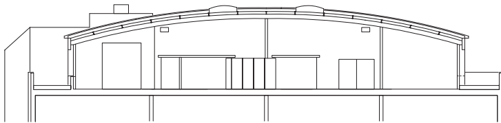
QUERSCHNITT GROSSRAUMBÜRO
