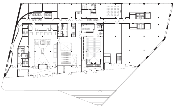
Plan +1 Maison des Religions
