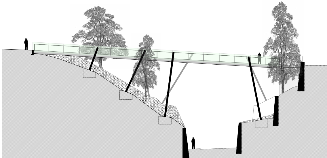
Elévation sud
