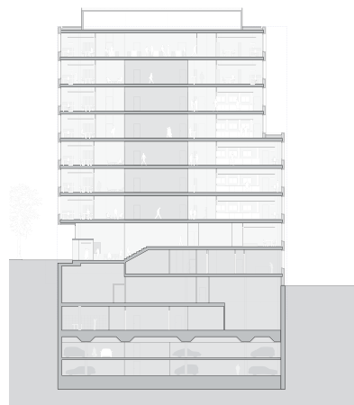
Coupe transversale
