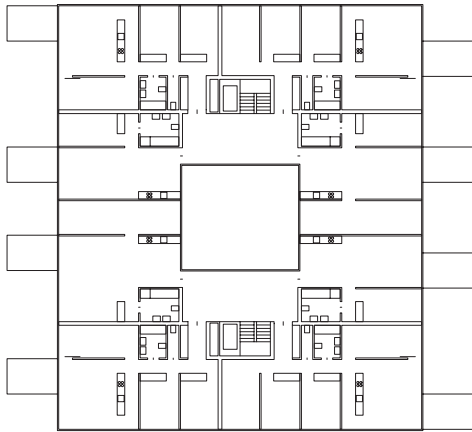
PLAN 1ER ETAGE | LES APPARTEMENTS SE DÉCLINENT AUTOUR D'UN PUIT DE LUMIÈRE CENTRAL ENTOURÉ DE PAROIS MATTES VITRÉES
