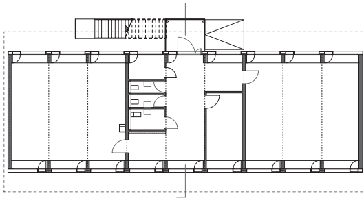
PLAN REZ-DE-CHAUSSÉE
