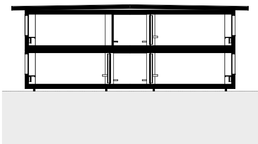
Querschnitt
