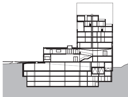
Schnitt
