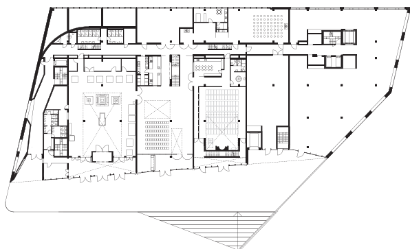
Grundriss +1 Haus der Religionen
