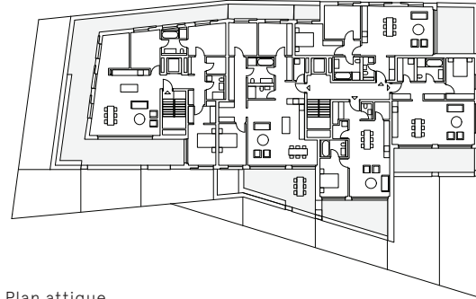
Plan attique
