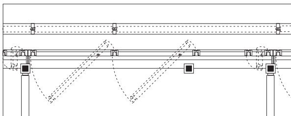
NOUVELLE FAÇADE AVEC DES OU- VERTURES À BATTANTS POUR UNE UTILISATION OPTIMALE DE LA LU- MIÈRE DU JOUR ET DES CLAPETS POUR LA VENTILATION NOCTURNE PASSIVE. STORES EXTÉRIEURS
